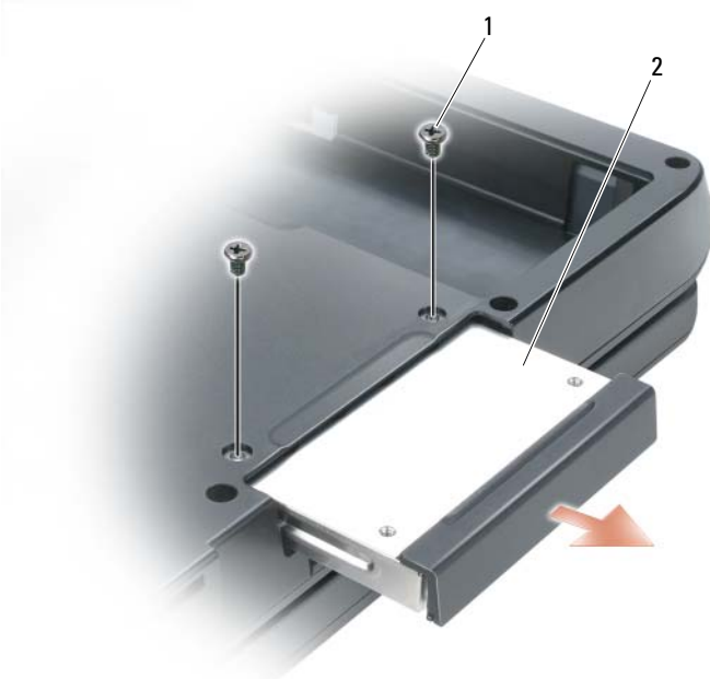
1 하드 드라이브 나사 (2 개 ) 2 하드 드라이브
