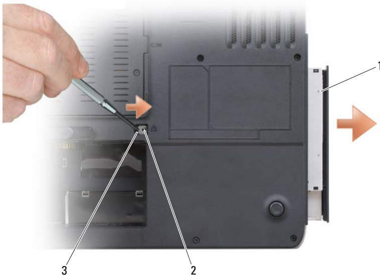
1 광학 드라이브 2 장치 고정 나사 3 노치
